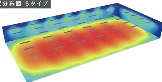
照度分布図 Sタイプ
